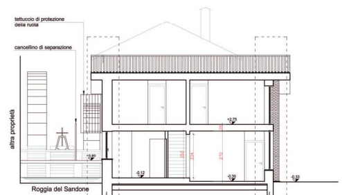
SEZIONE PROGETTO 02
