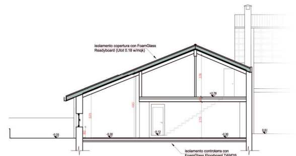
SEZIONE PROGETTO 01
