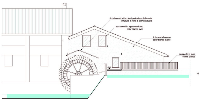
PROSPETTO PROGETTO 03
