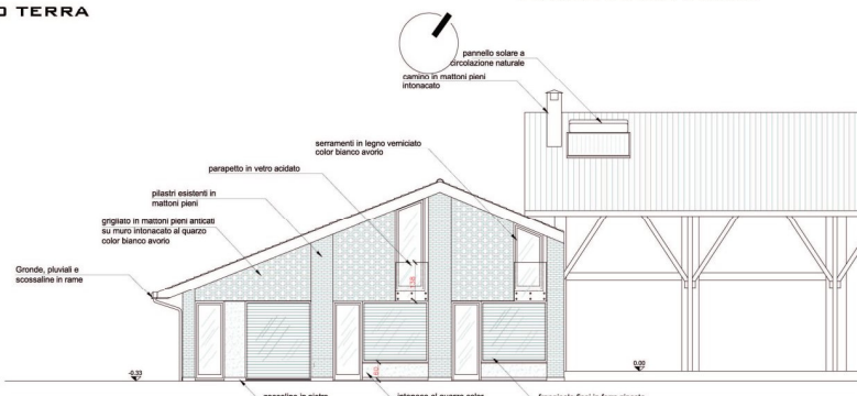
PROSPETTO PROGETTO 01
